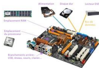
Carte mère
